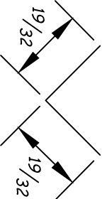
BOTTOM VEE
